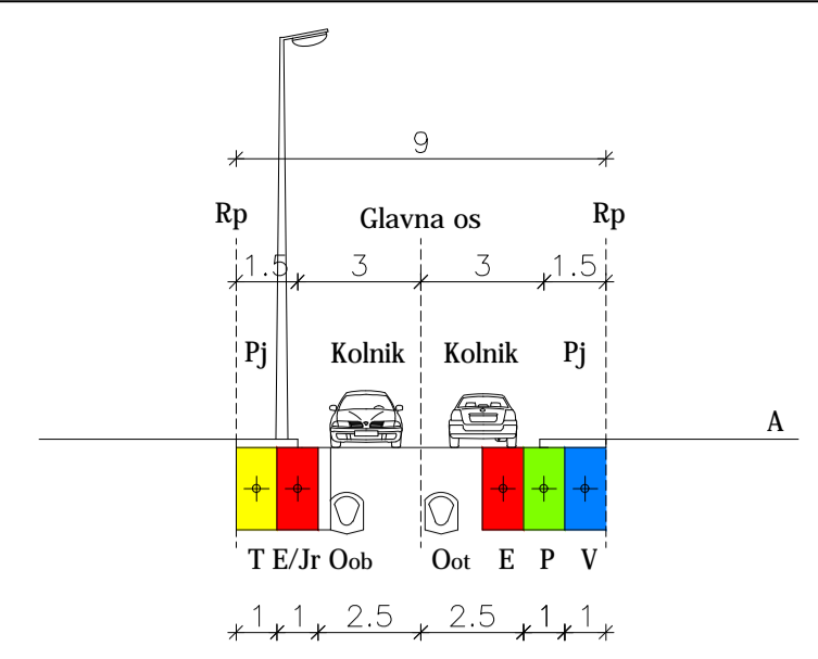
POPREČNI PROFIL PLANIRANE ULICE 'A' I 'B' - m.1:200
