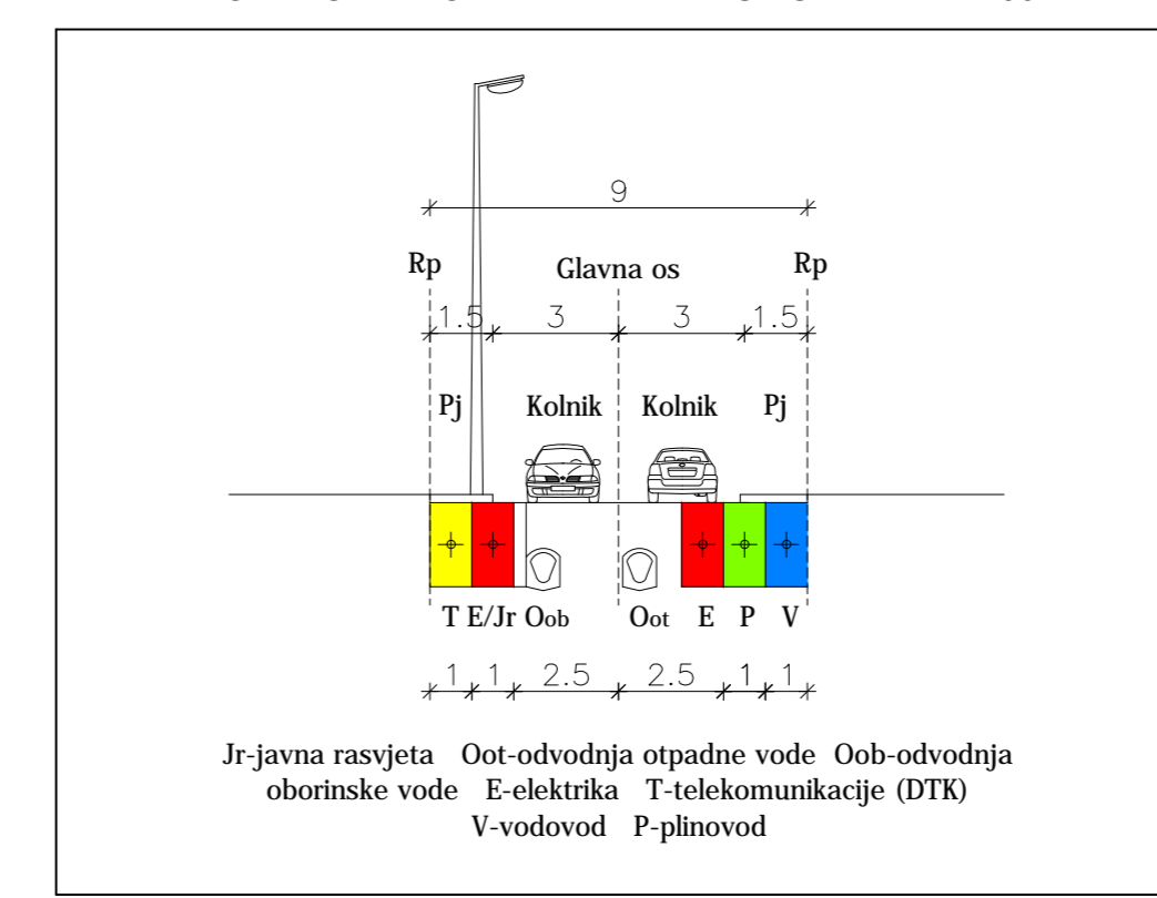
POPREČNI PROFIL PLANIRANE ULICE 'A' - m.1:200
