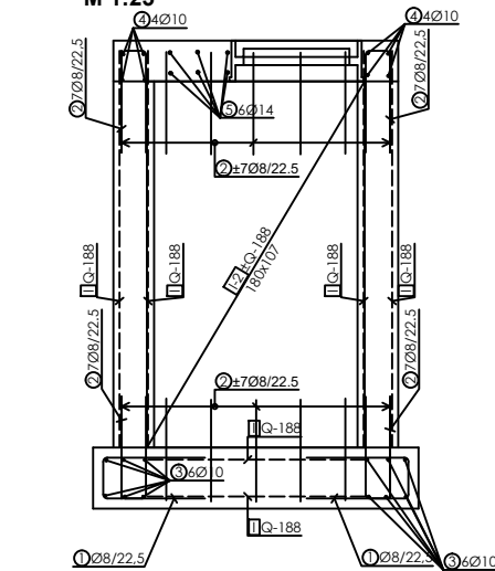
TEMELJNA PLOČA - TLOCRT / M 1:25
