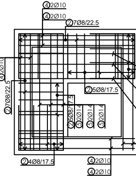
PLOČA OKNA - TLOCRT / M 1:25
