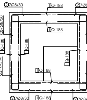
PLOČA OKNA - TLOCRT / M 1:25
