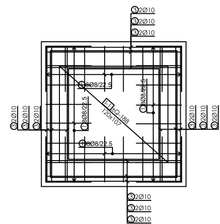
TEMELJNA PLOČA - TLOCRT / M 1:25
